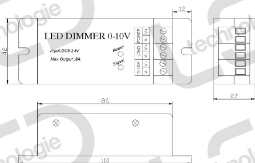
rozměry v mm
