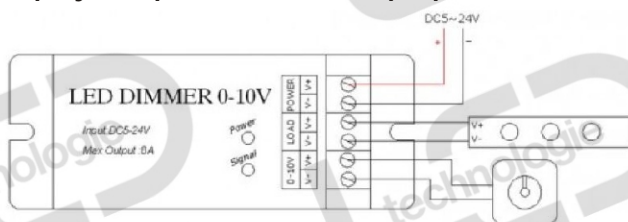
zapojení stmívače
